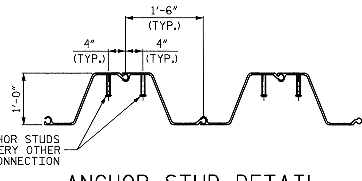
ANCHOR STUD DETAIL
