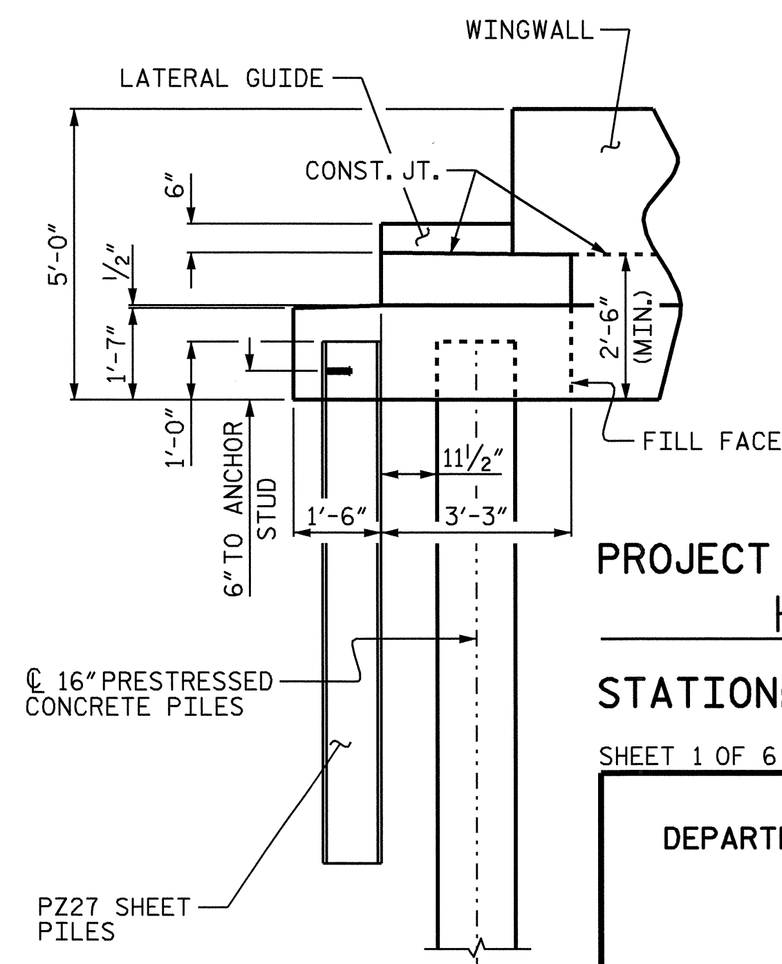
END ELEVATION
