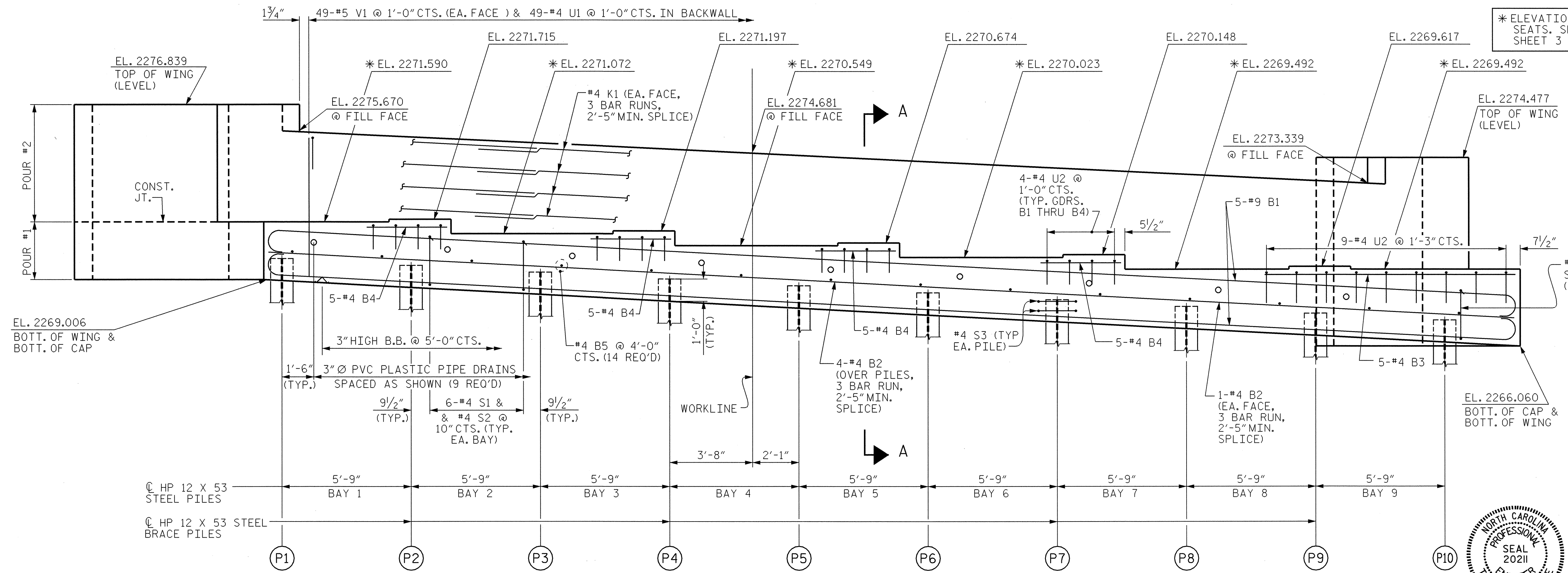
ELEVATION
