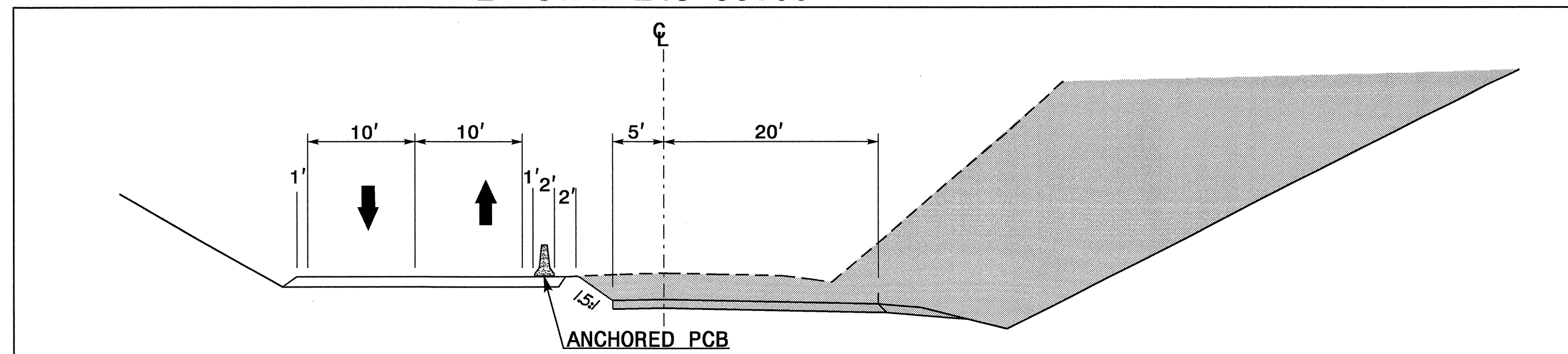
SECTION B-B' -L- STA. 243+50.00
