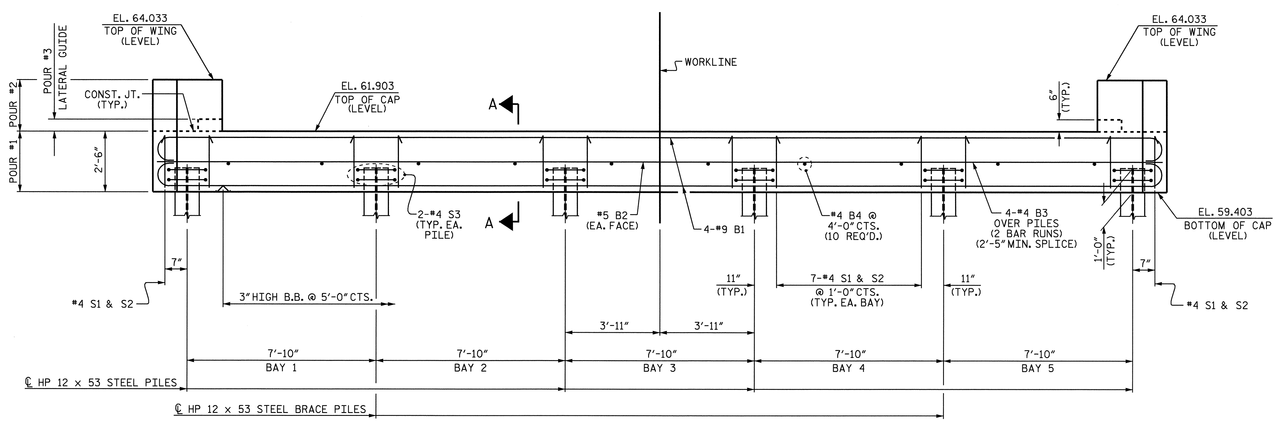
ELEVATION
