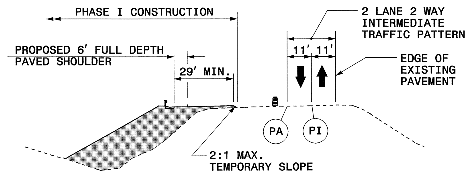
SECTION K-K' (STA. 168+00 +/- -L-)
