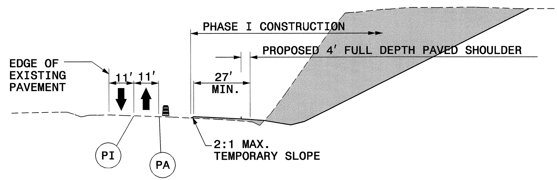
SECTION L-L' (STA. 195+00 +/- -L-)
