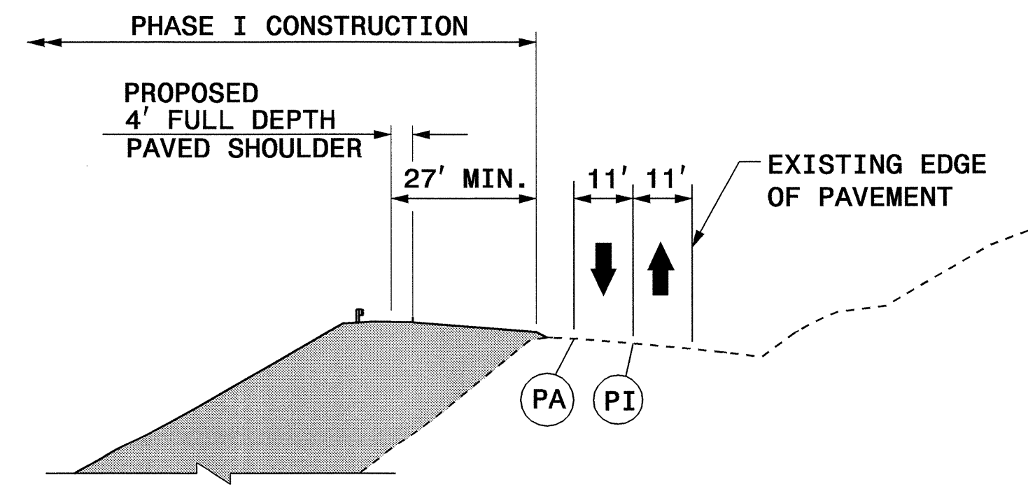
SECTION P-P' (STA. 270+00 +/- -L-)
