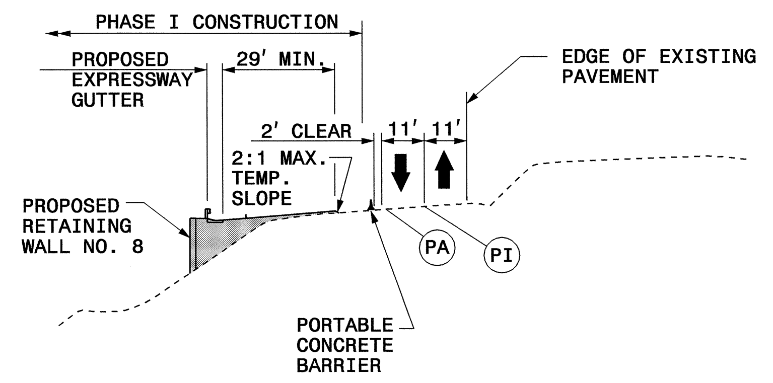
SECTION U-U' (STA. 345+50 +/- -L-)
