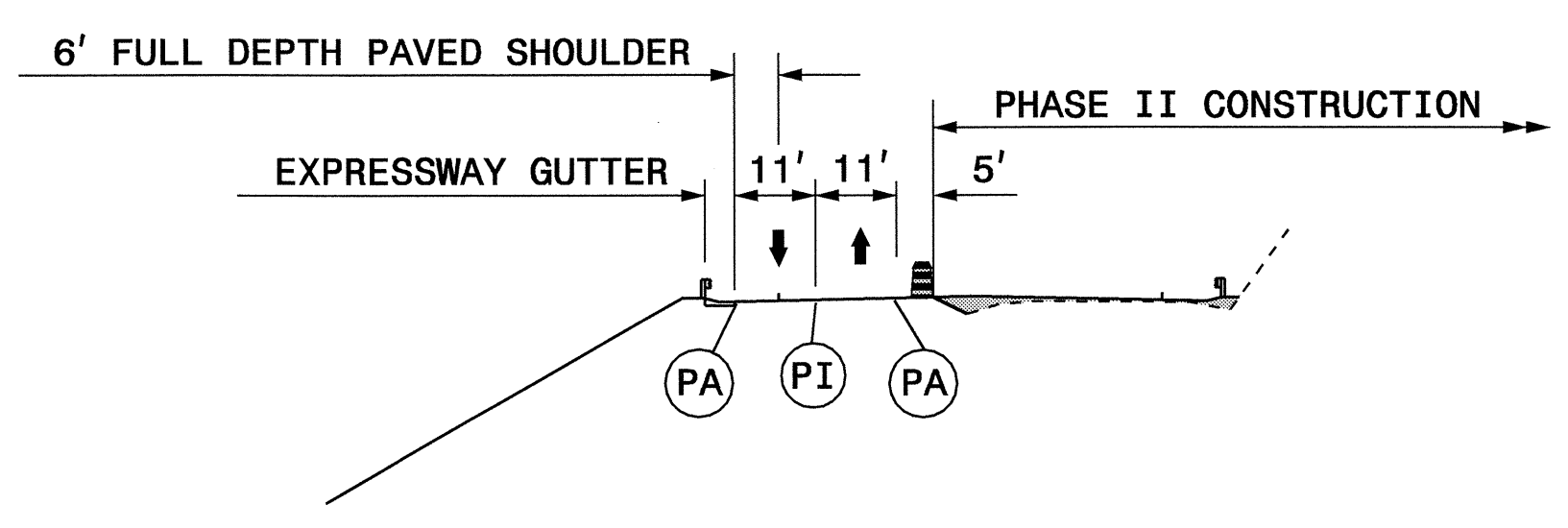
SECTION CC-CC' (STA. 50+00 +/- -L-)
