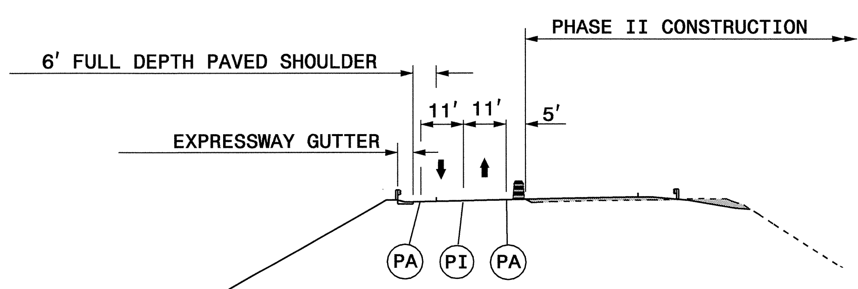
SECTION JJ-JJ' (STA. 169+00 +/- -L-)
