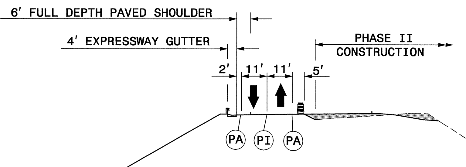
SECTION 00-00' (STA. 264+00 +/- -L-)
