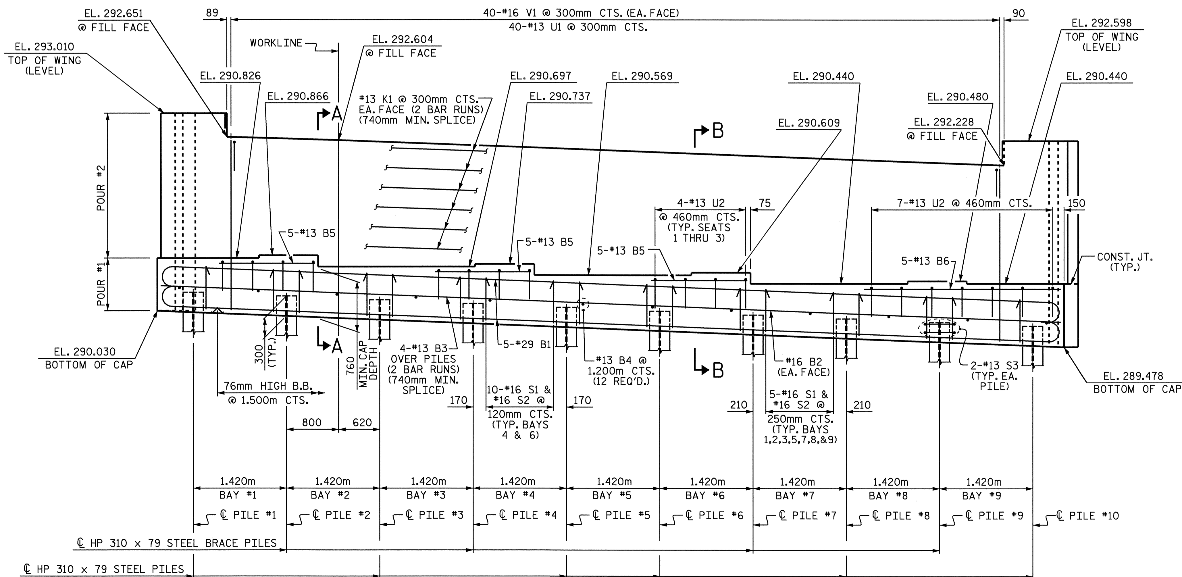
ELEVATION
