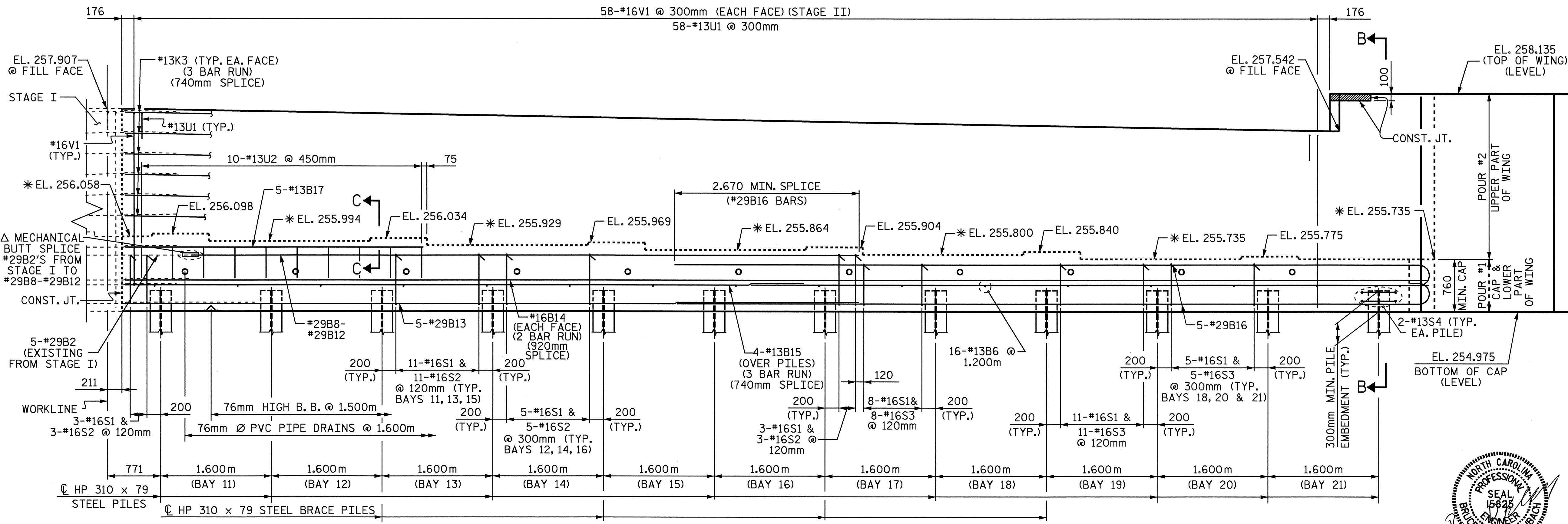
ELEVATION
