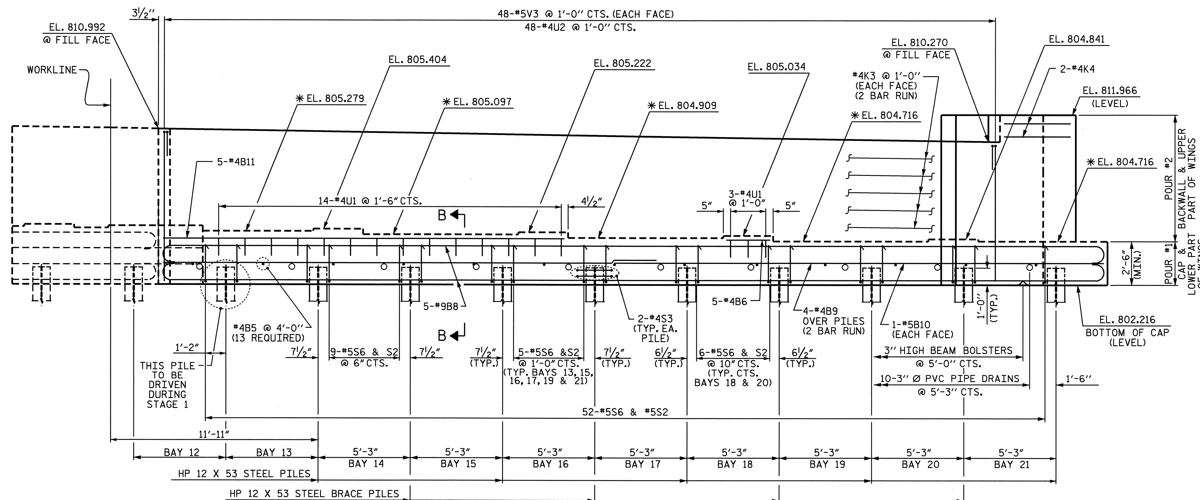
ELEVATION
