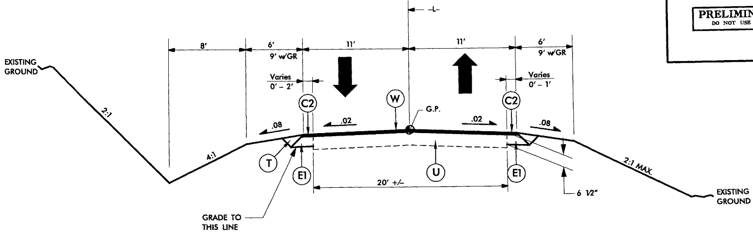
TYPICAL SECTION NO. 1 -L- STA 15+25 TO -L- STA 18+00 -L- STA 20+00 TO -L- STA 22+50
