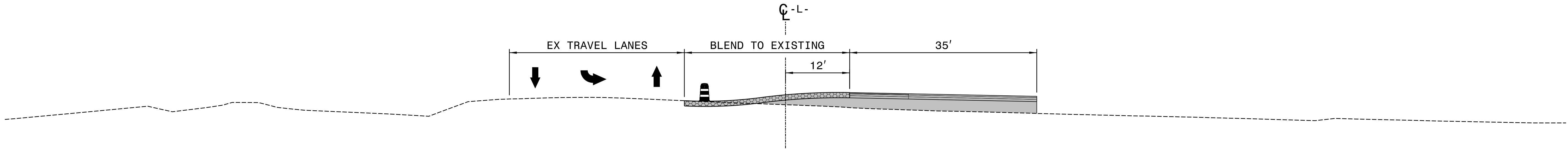
SECTION AS-AS
