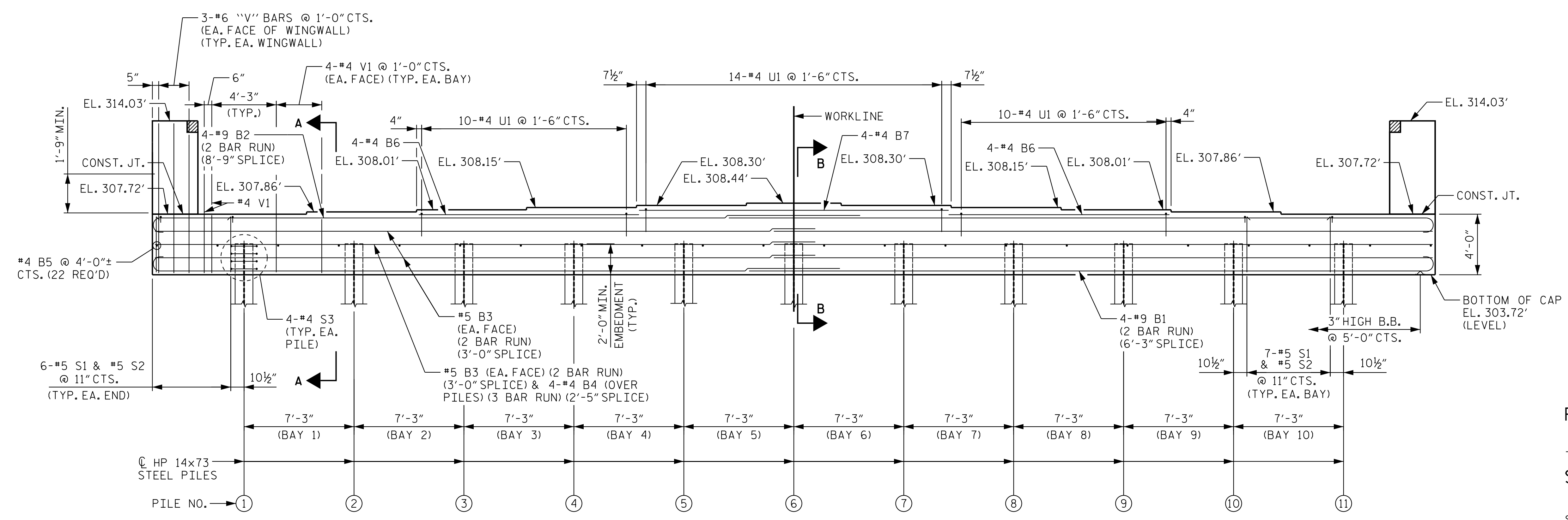
ELEVATION
