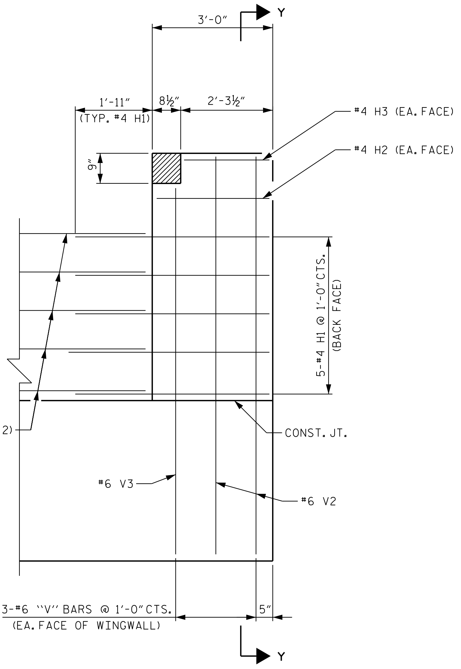
ELEVATION
