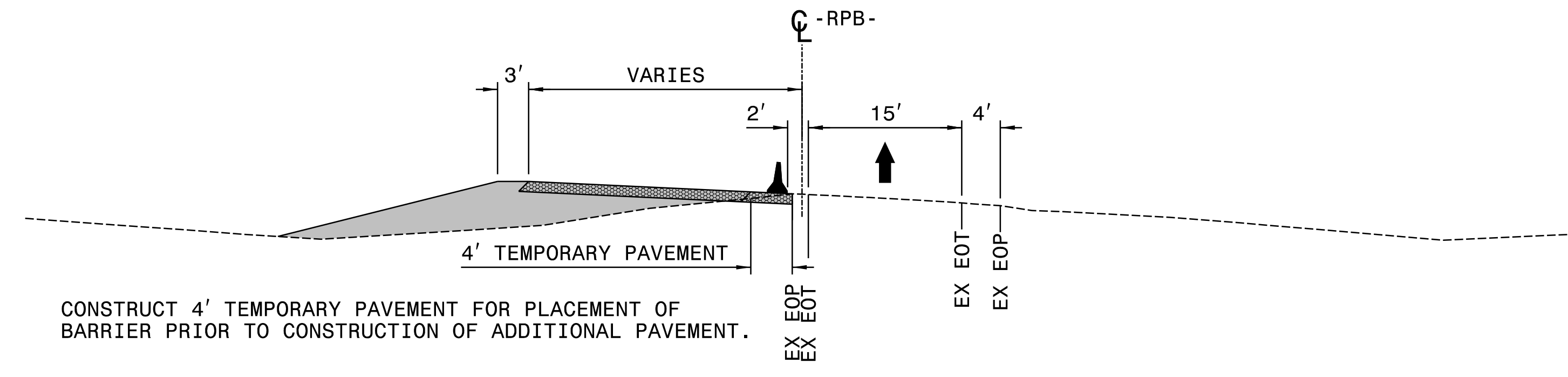
SECTION D-D
