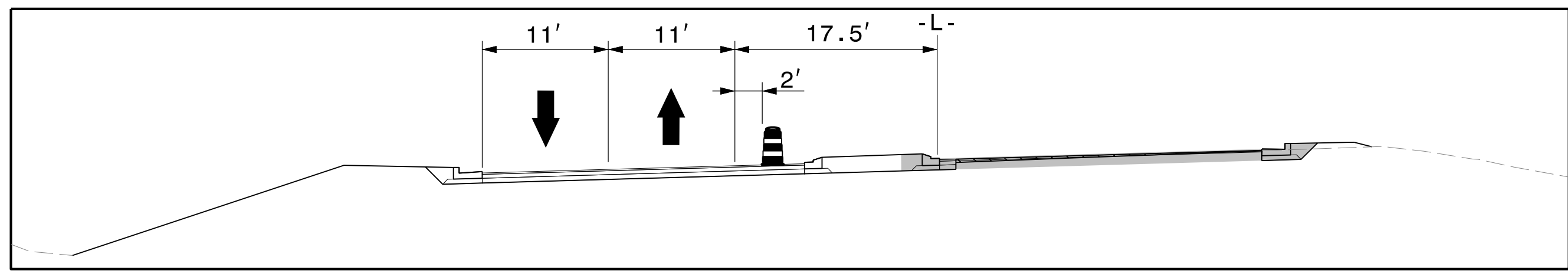
A-A STA. 20+50
