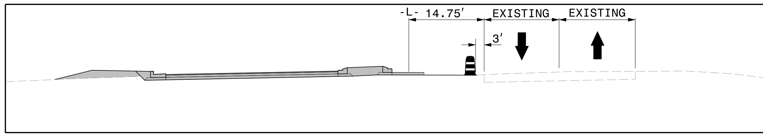
A-A STA. 22+00
