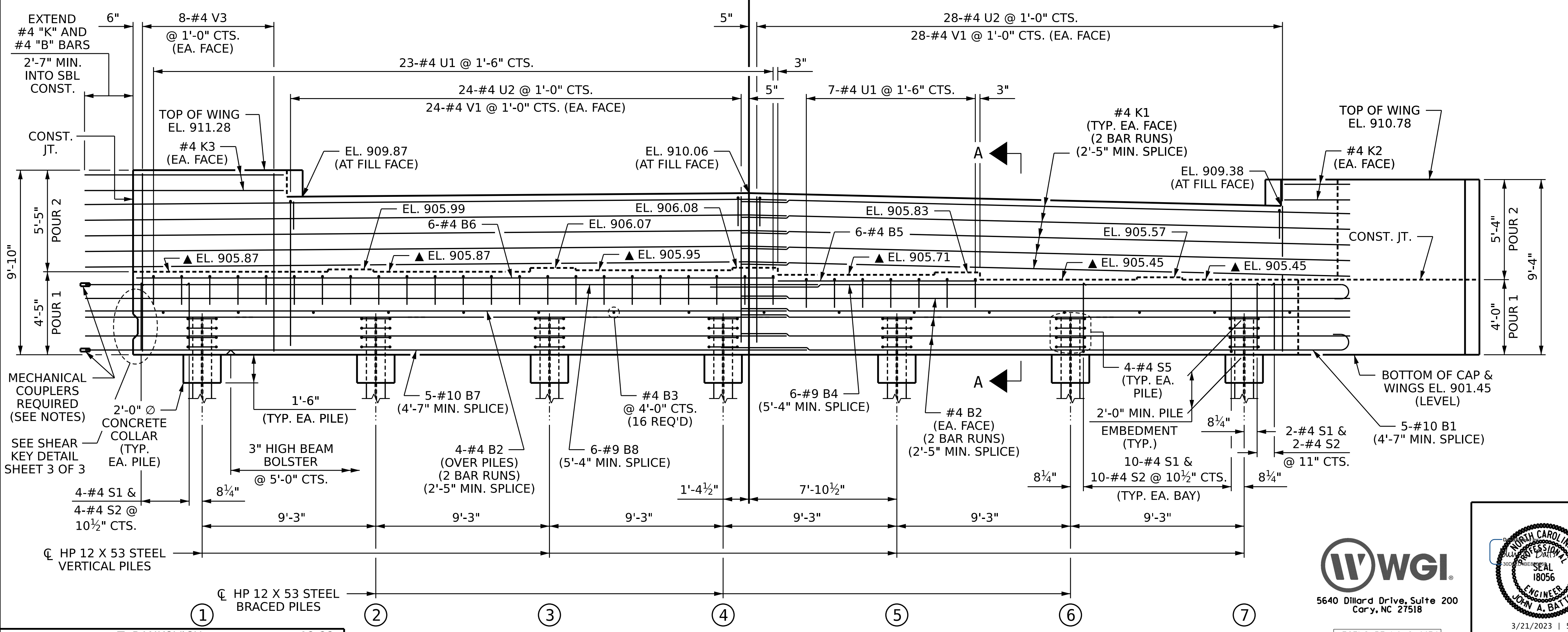
ELEVATION
