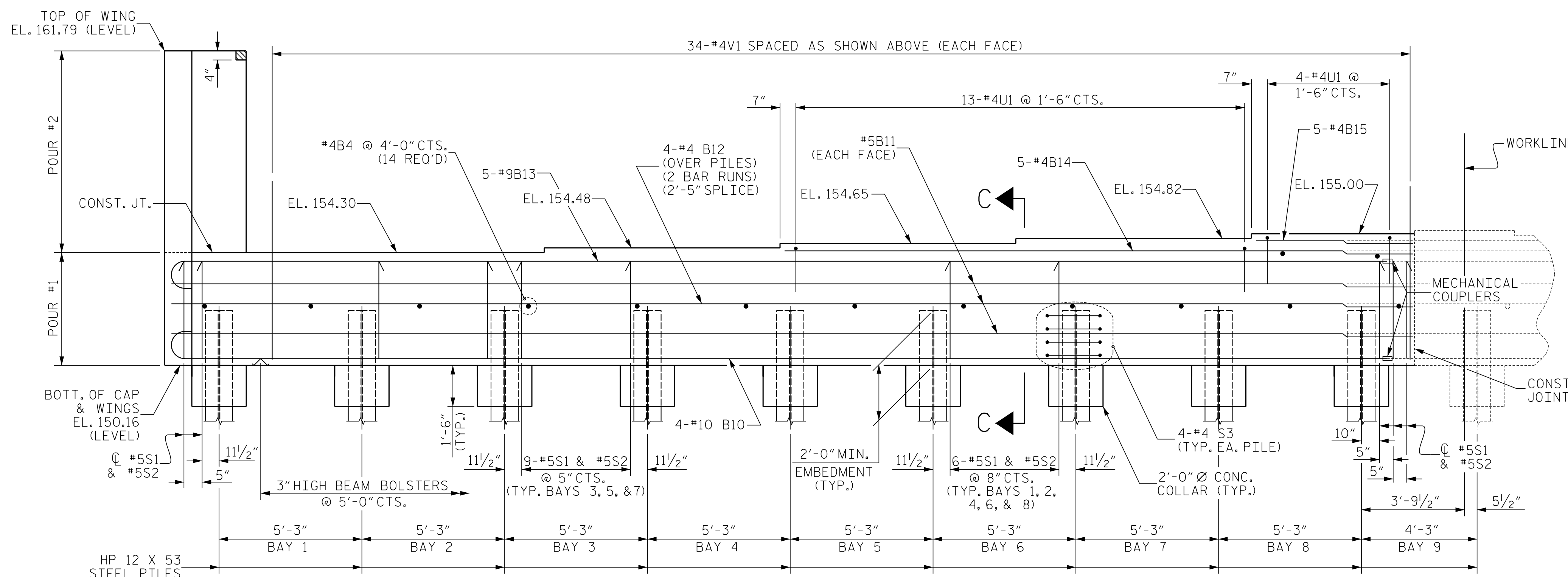
ELEVATION
