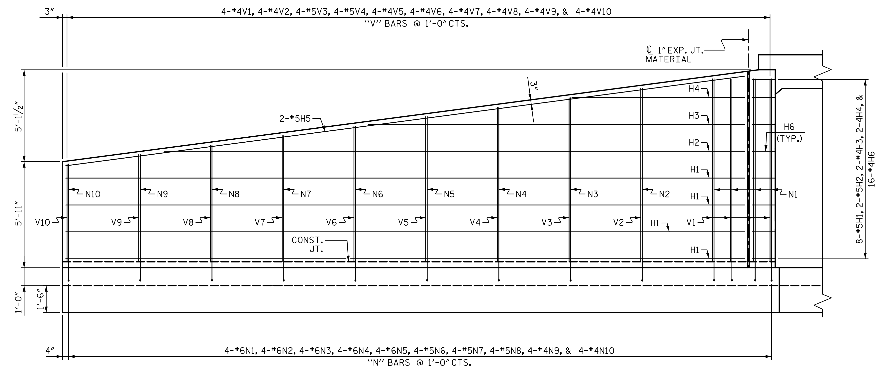
ELEVATION W1
