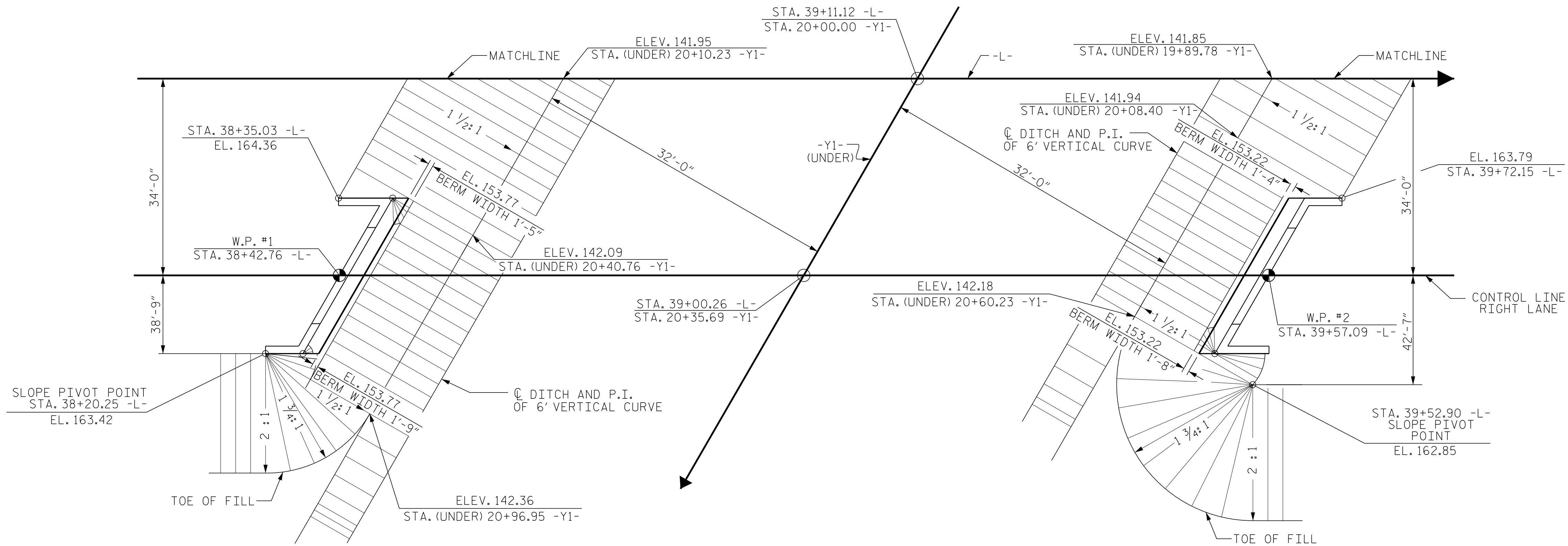
END BENT 1
