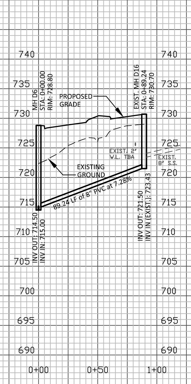
SANITARY SEWER PROFILE 8" SEWER LINE D2 - MH D6 to MH D16 STA. 0+00 to 0+89.24
