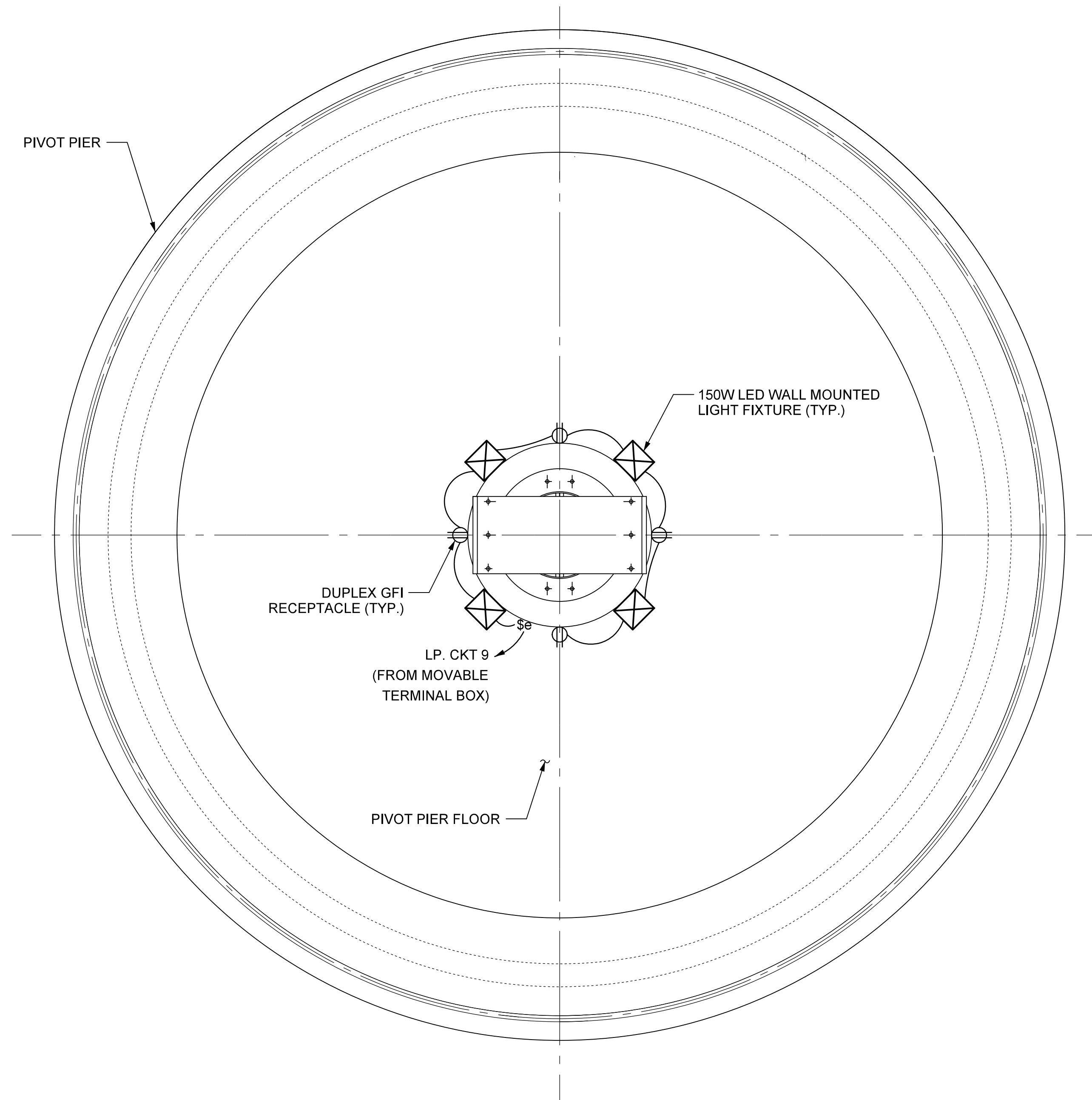
PIVOT PIER LAYOUT SCALE: 3/8" = 1'-0"
