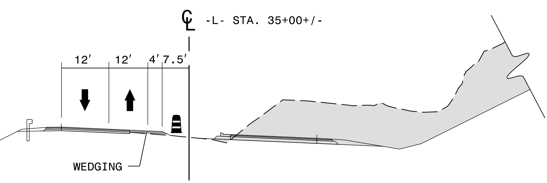
SECTION D-D
