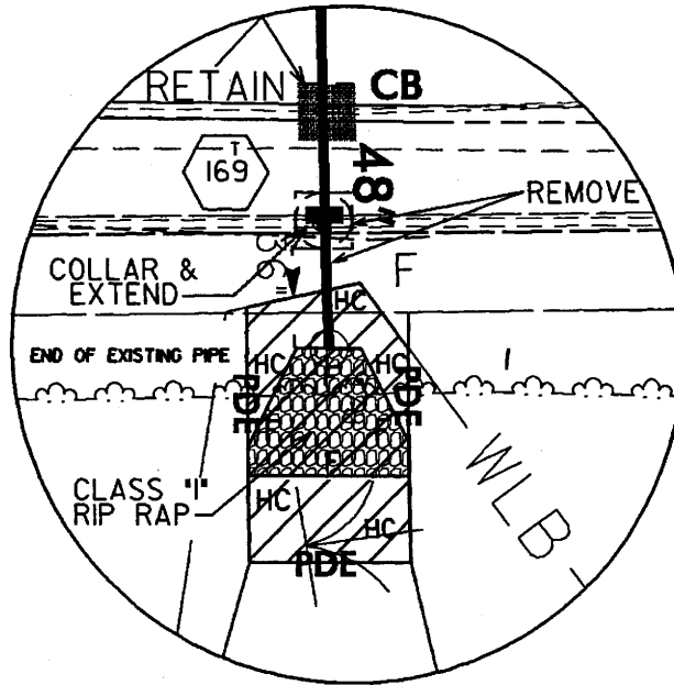
ENLARGEMENT, SITE 3
