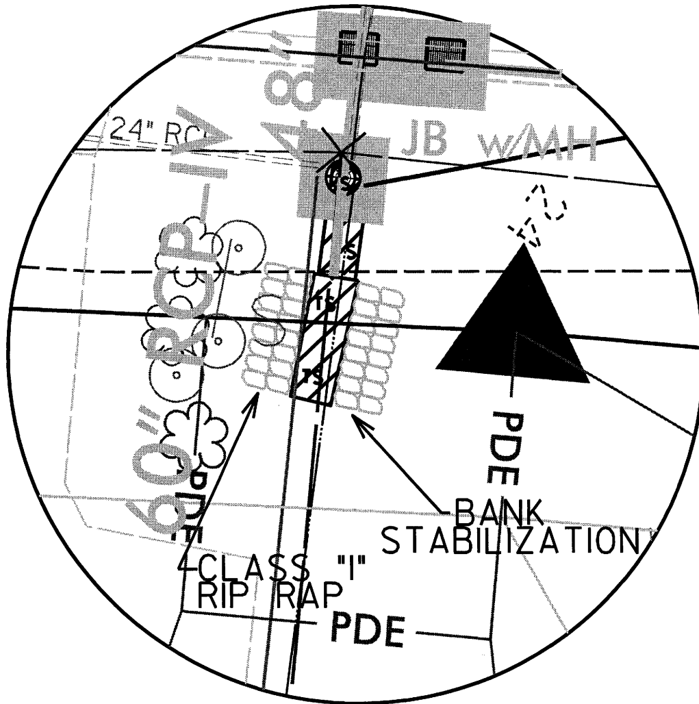
ENLARGEMENT, SITE 1
