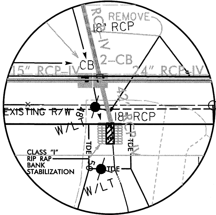
ENLARGEMENT, SITE 2
