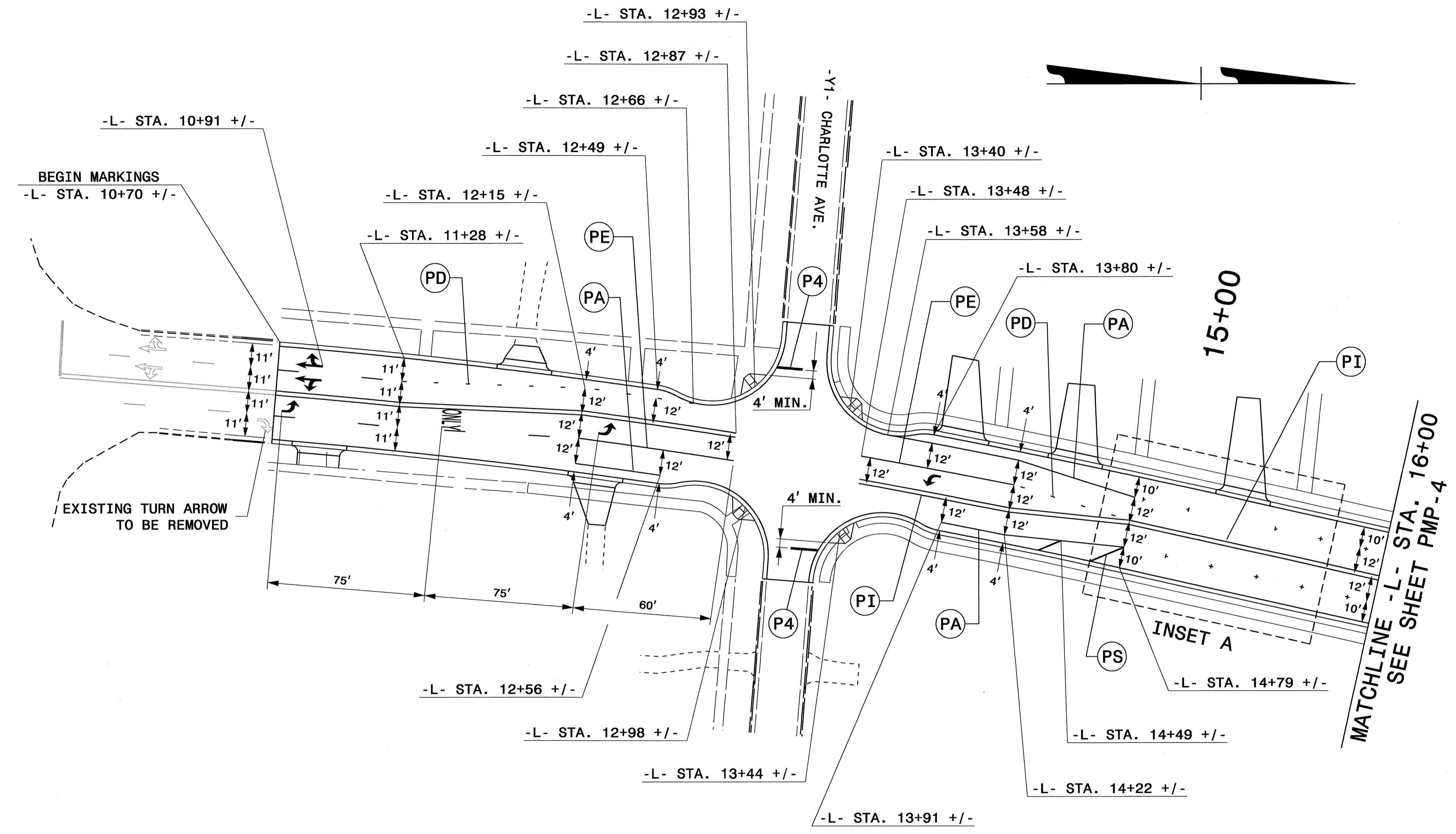
INSET A
