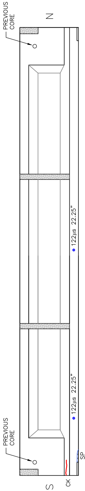
G2—East Elevation
