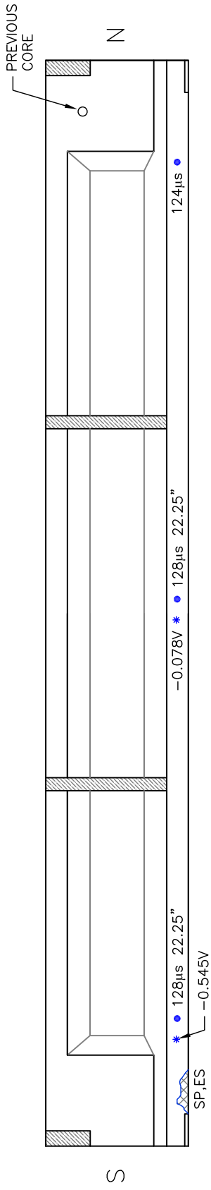
G3—East Elevation
