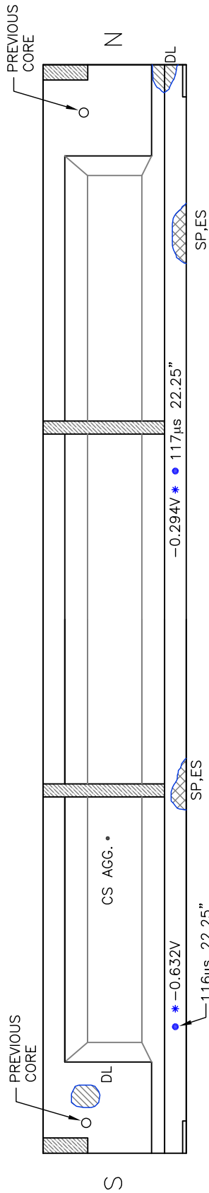
G3—East Elevation
