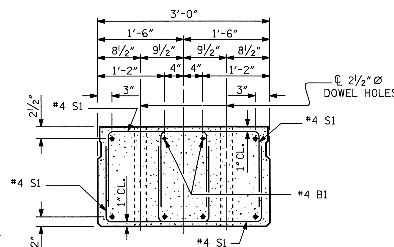
END ELEVATION
