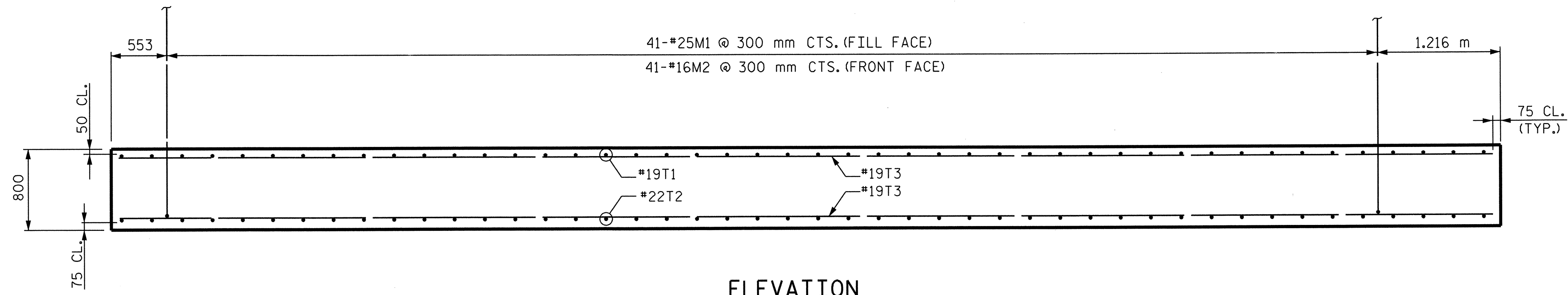
ELEVATION
