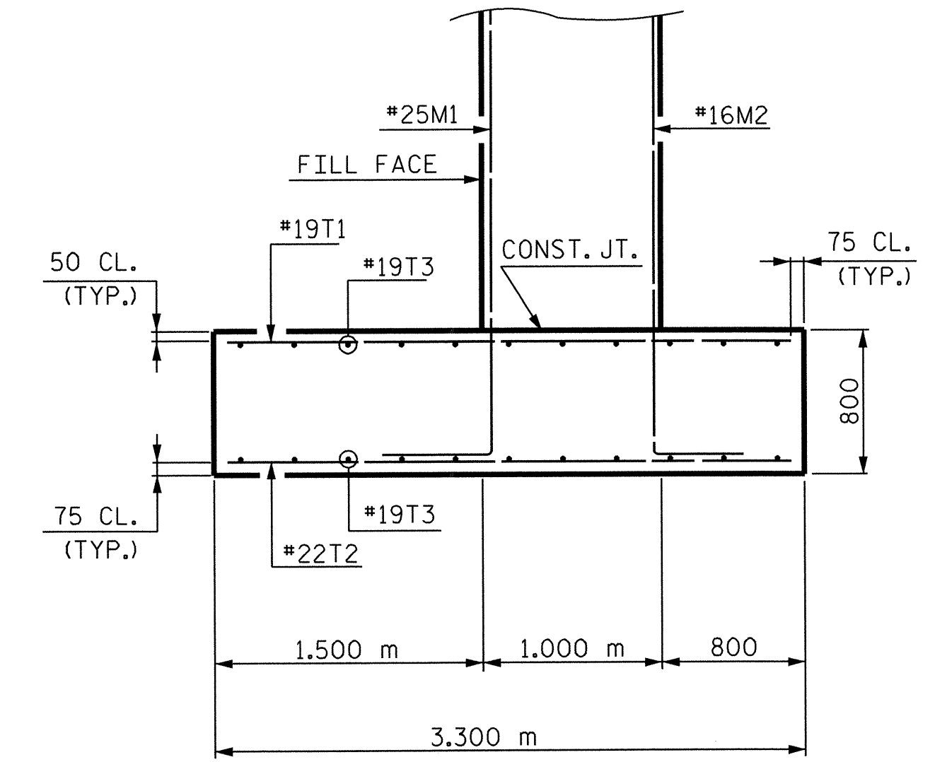
SECTION A-A
