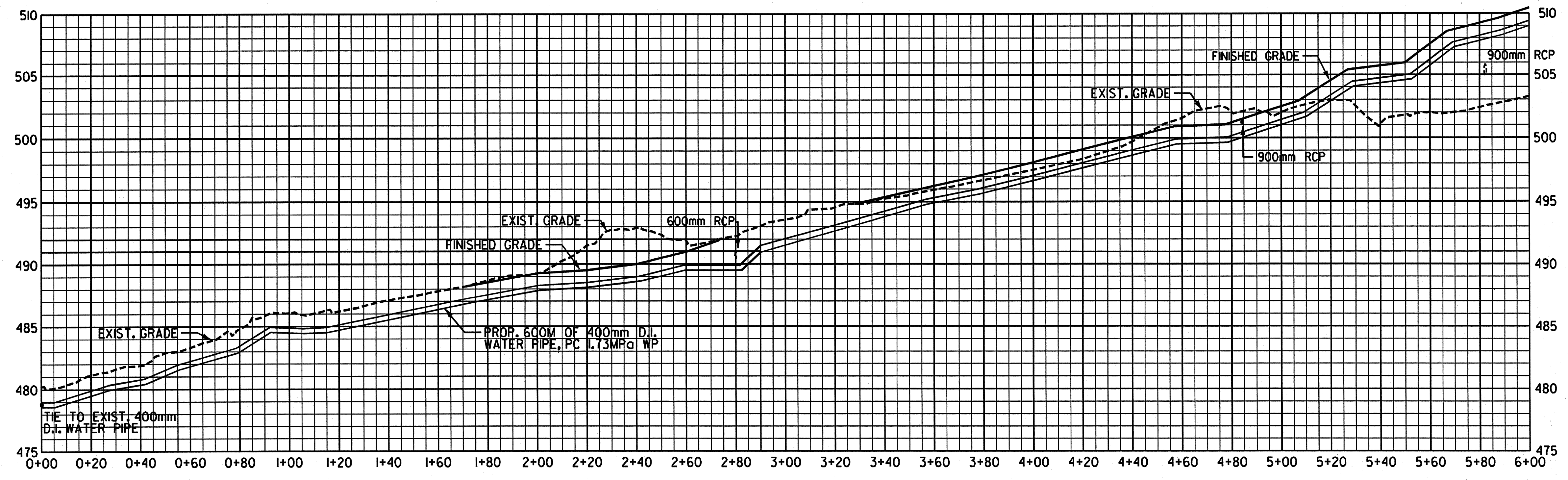
LINE 3 SCALE: HORIZ.: 1=1000 VERT.: 1=200
