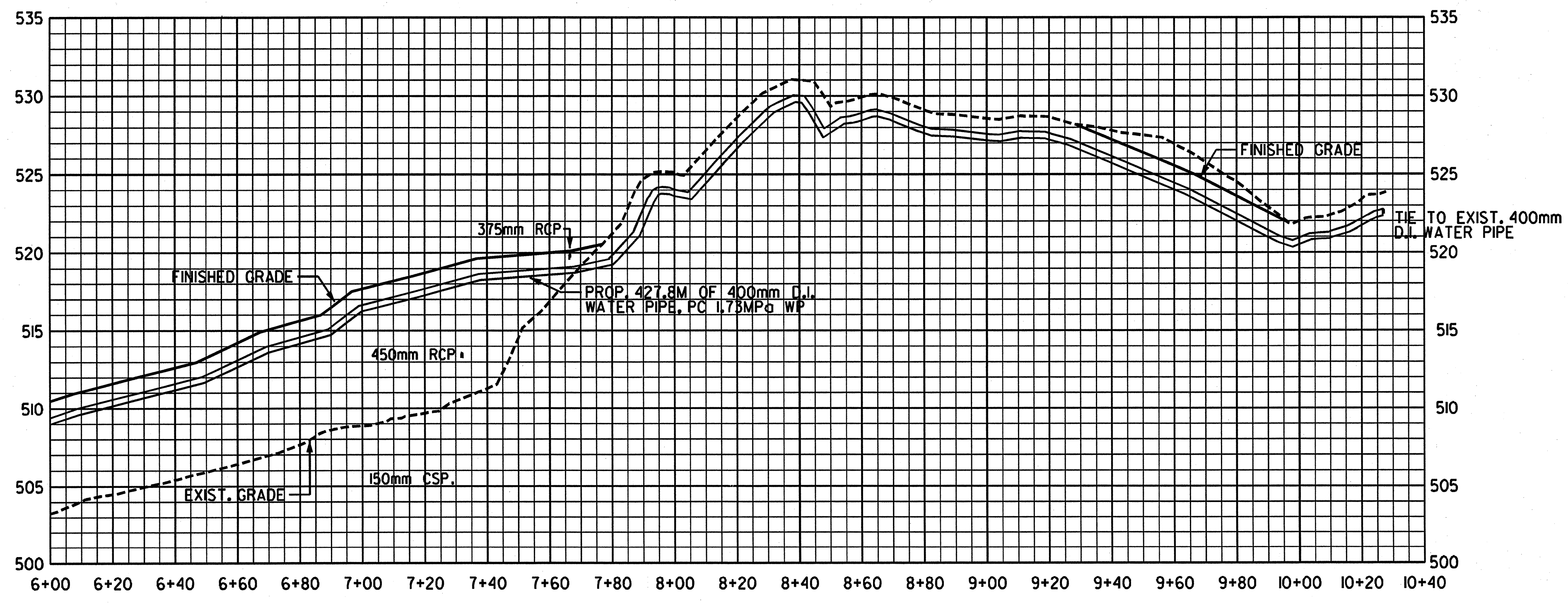
LINE 3 SCALE: HORIZ.: 1=1000 VERT.: 1=200
