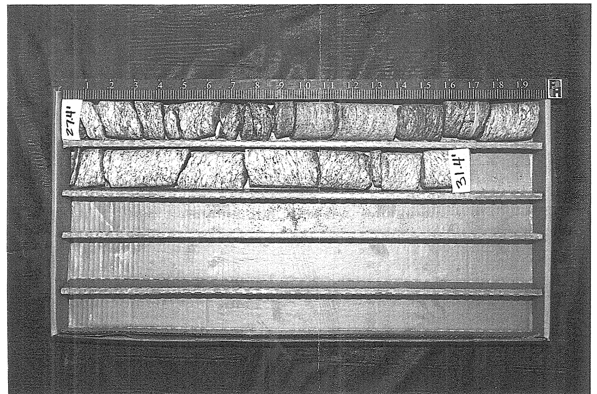
BORING EB2-A STA. 14+85 -L- @ 15.0 LEFT BOX 2 of 2
