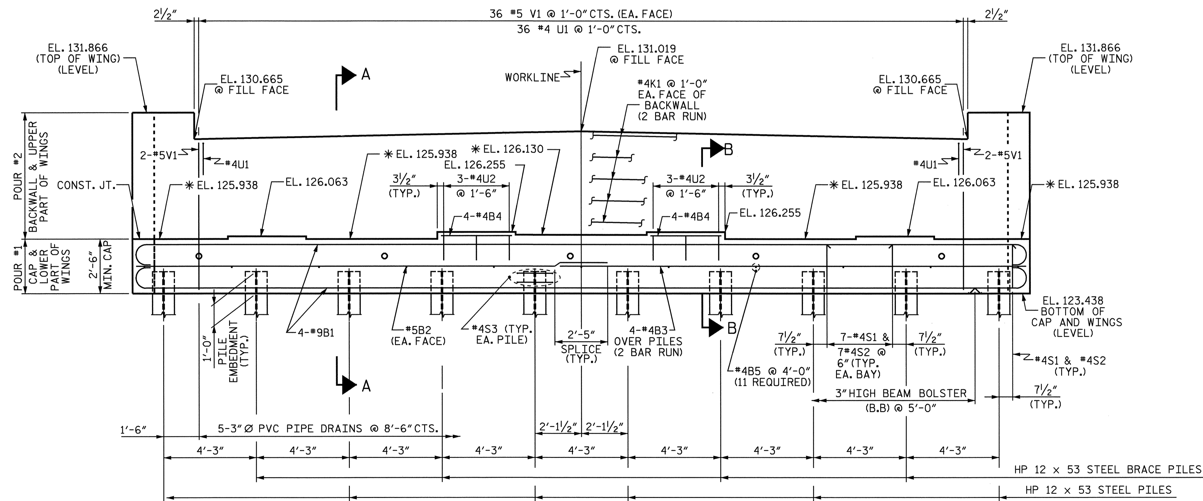
ELEVATION
