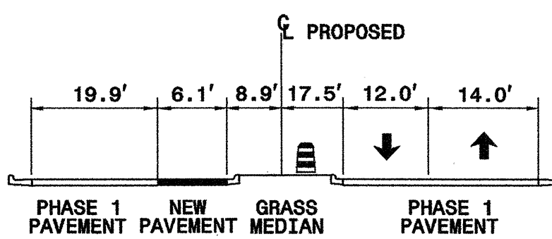
SECTION A-A -L- STA 20+00
