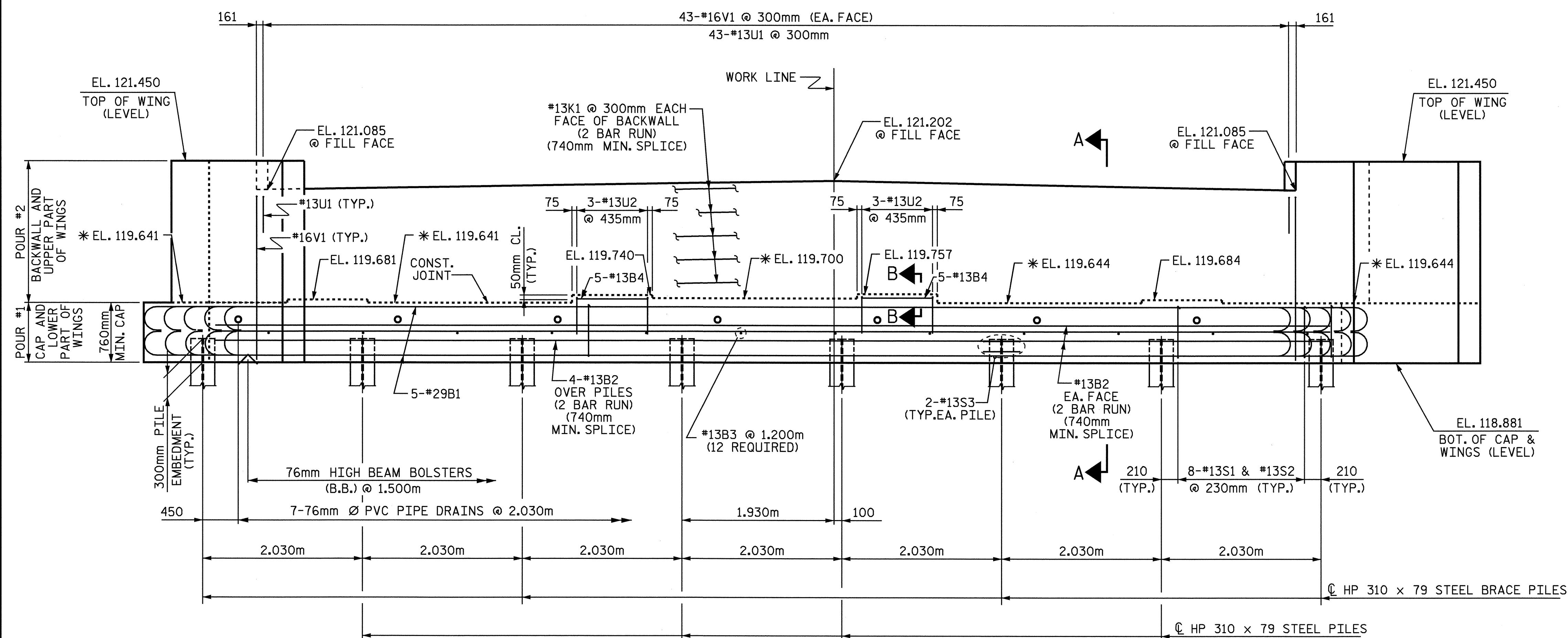
ELEVATION
