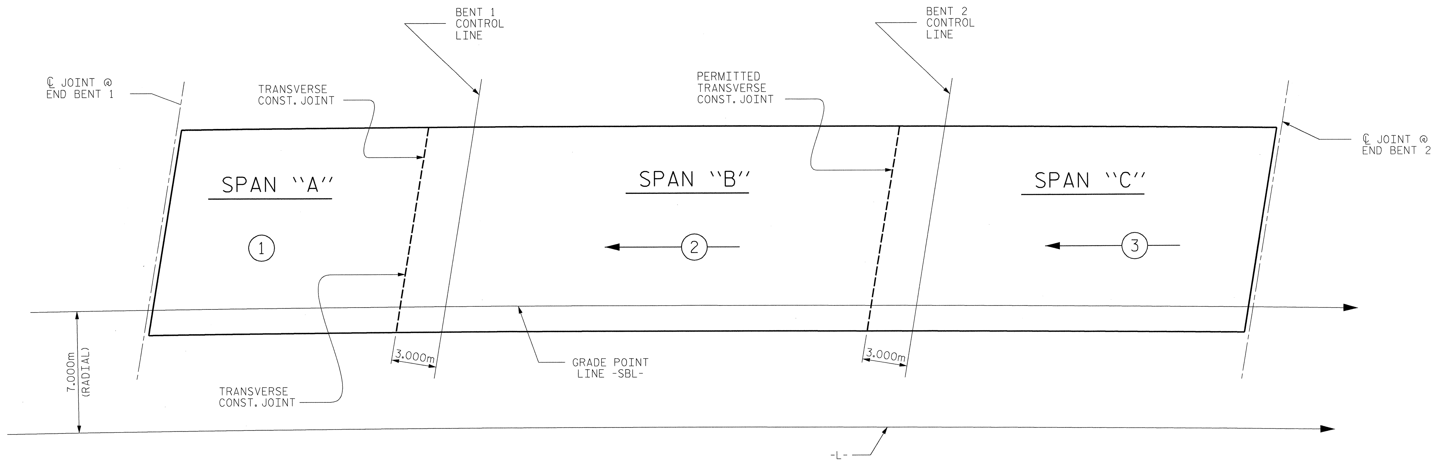
POUR SEQUENCE
