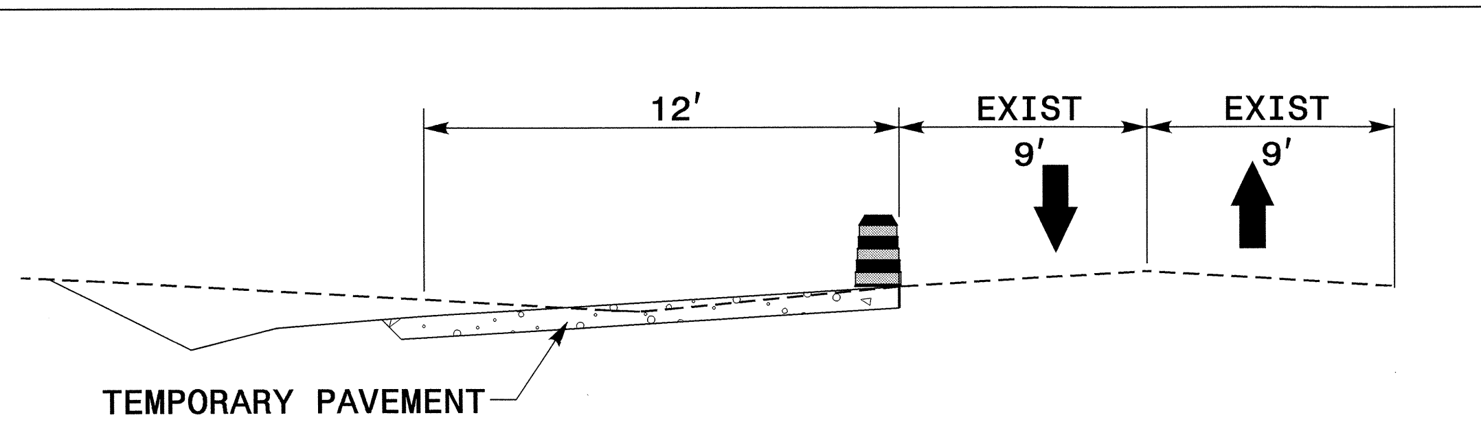
SECTION A-A -L- STA 28+50 +/-
