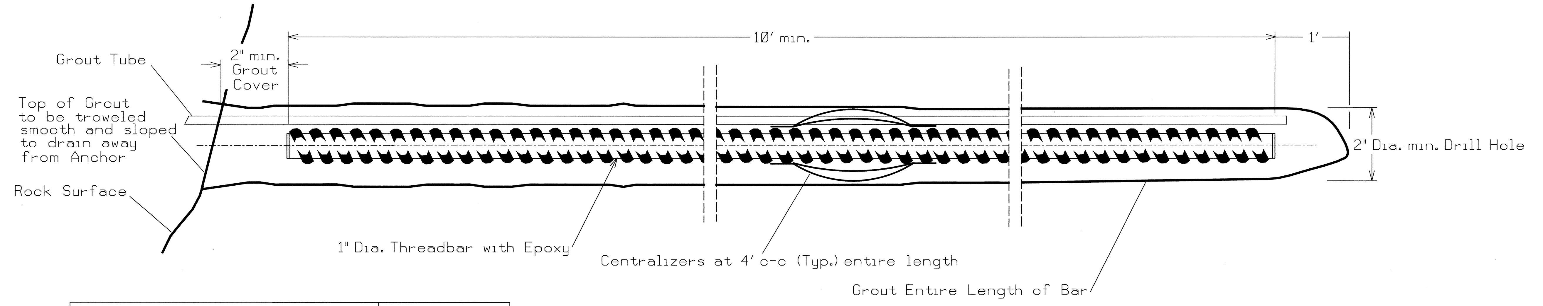
Tensioned Rock Bolt - Type II N. T. S.
