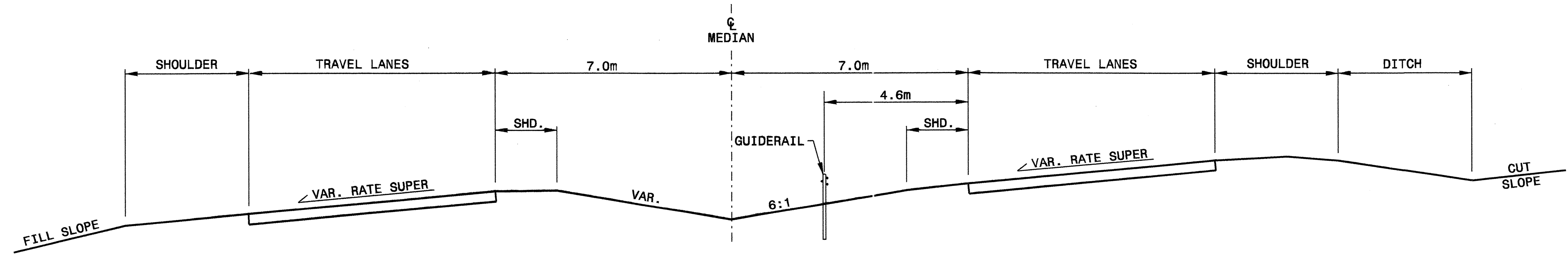
SECTION A-A
